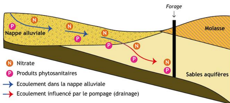
Figure 11 : Représentation schématique de l'inversement du sens d'écoulement d'une nappe alluviale libre sous l'effet d'un pompage réalisé les nappes captives (sables aquifères).
