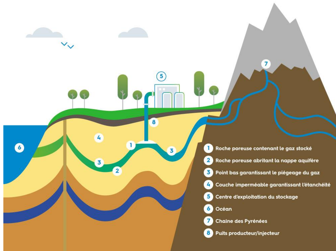
Figure 9: Représentation schématique des sites de stockage de gaz (source Terega).
